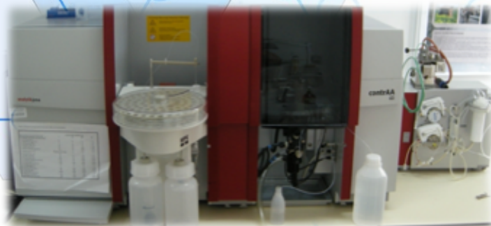
Analytic Jena ContrAA700 AAS
